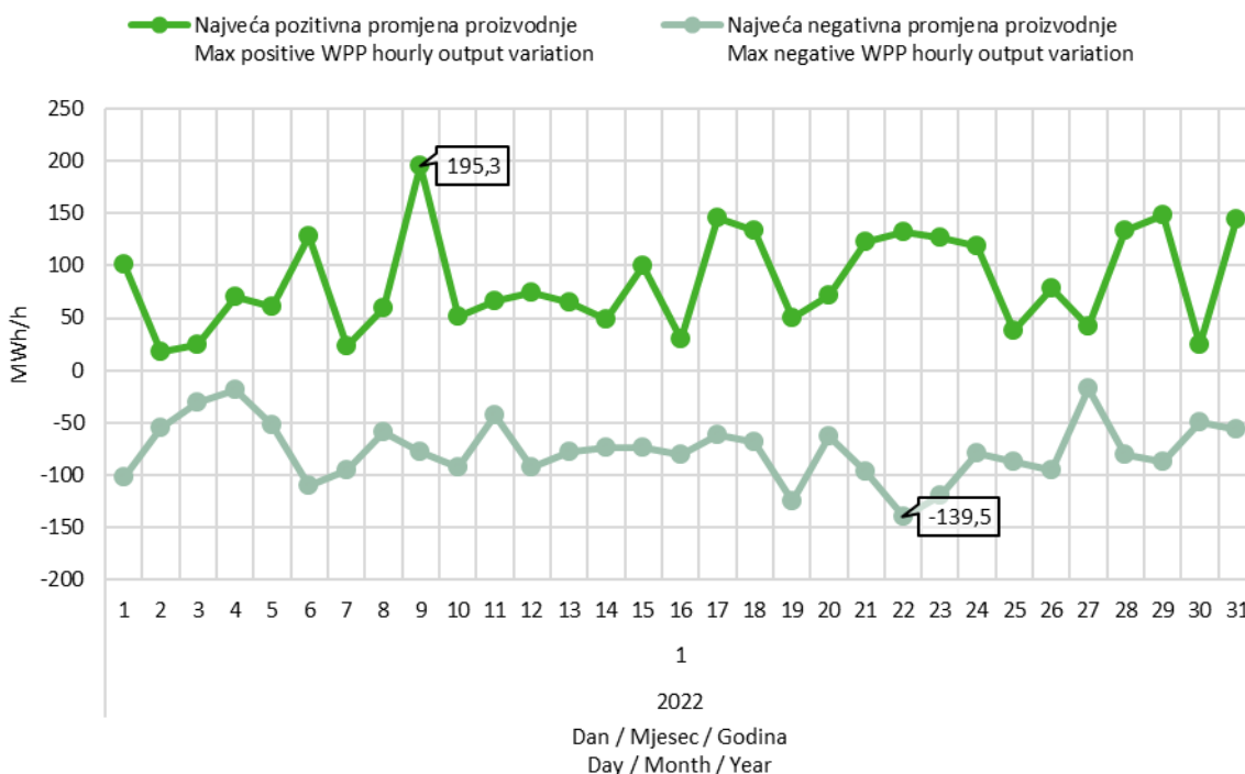
Slika 9 Maksimalna pozitivna i maksimalna negativna promjena satne proizvodnje VE u siječnju 2022. godine
