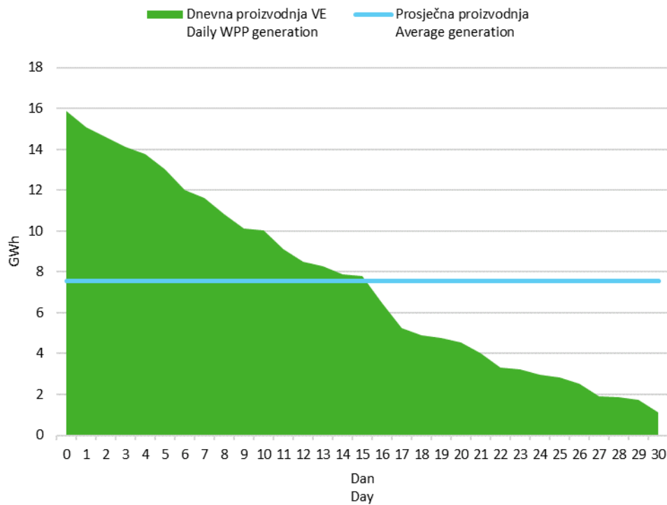
Slika 6 Krivulja trajanja dnevne proizvodnje vjetroelektrana u siječnju 2022. godine
