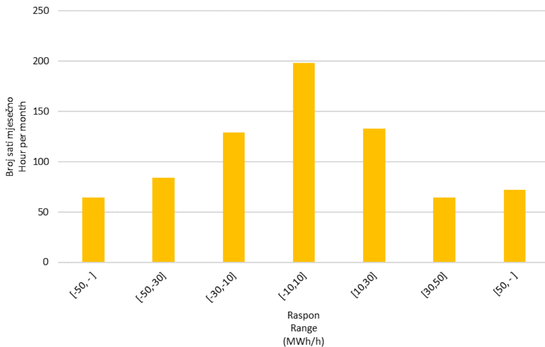
Slika 10 Statistička raspodjela satnih promjena proizvodnje VE u siječnju 2022. godine
