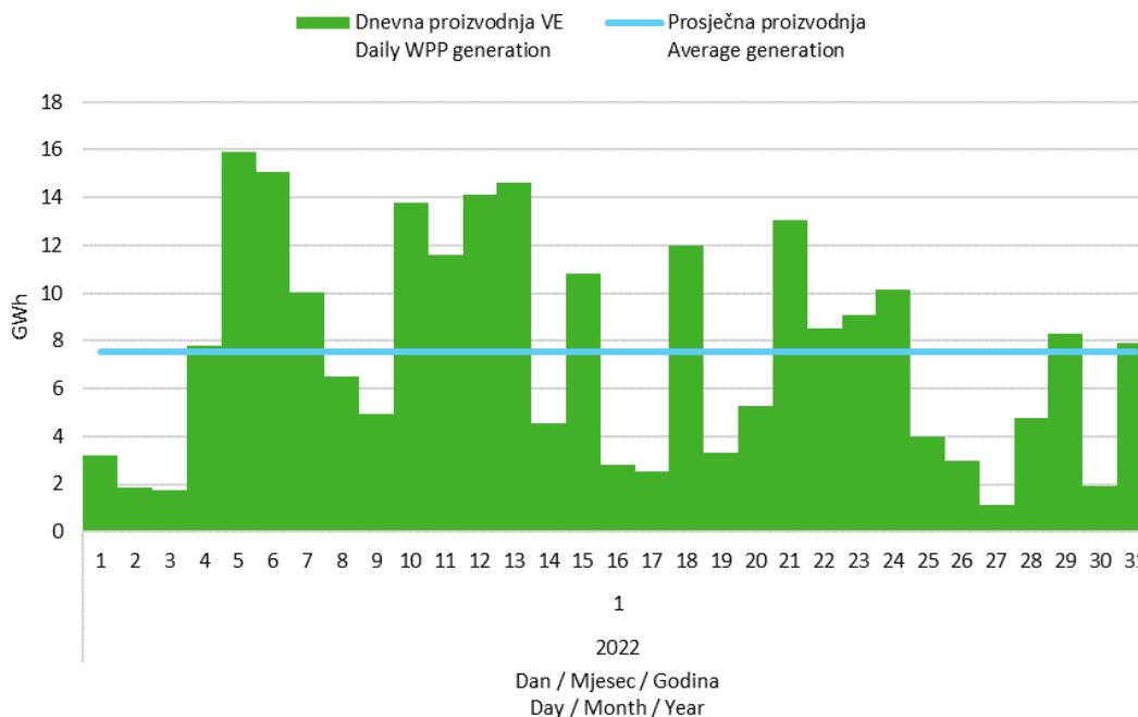
Slika 5 Dnevna proizvodnja svih vjetroelektrana u siječnju 2022. godine
