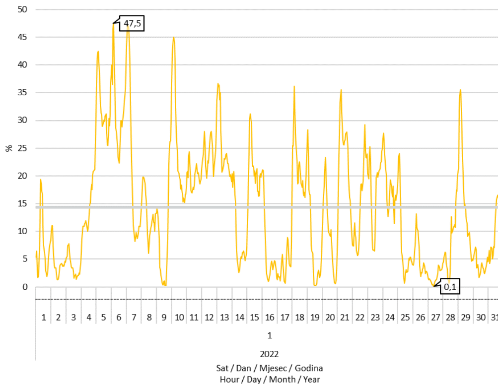
Slika 8 Udio proizvodnje vjetroelektrana u pokrivanju satnog opterećenja elektroenergetskog sustava u siječnju 2022. godine
