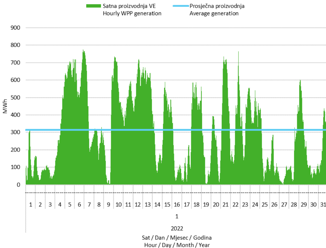
Slika 2 Satna proizvodnja svih vjetroelektrana u siječnju 2022. godine
