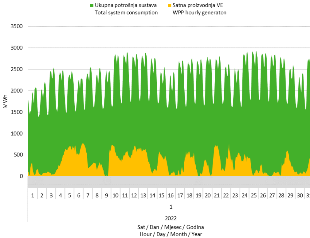
Slika 7 Usporedba satnog dijagrama opterećenja sustava i proizvodnje vjetroelektrana u siječnju 2022. godine
