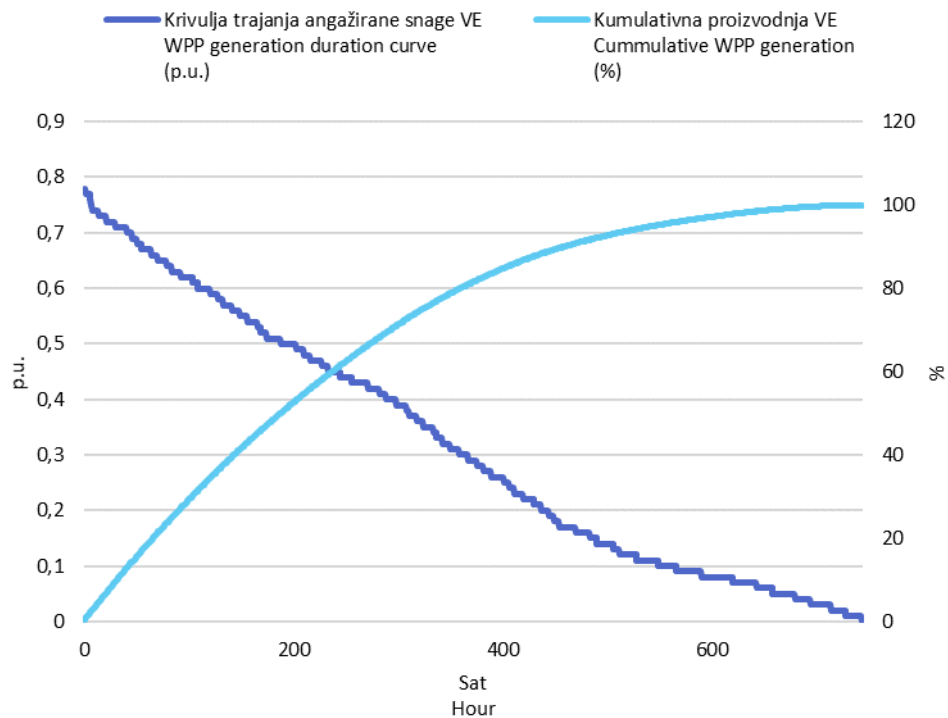
Slika 3 Krivulja trajanja angažirane snage svih VE i kumulativna proizvodnja VE u siječnju 2022. godine u jediničnim vrijednostima
